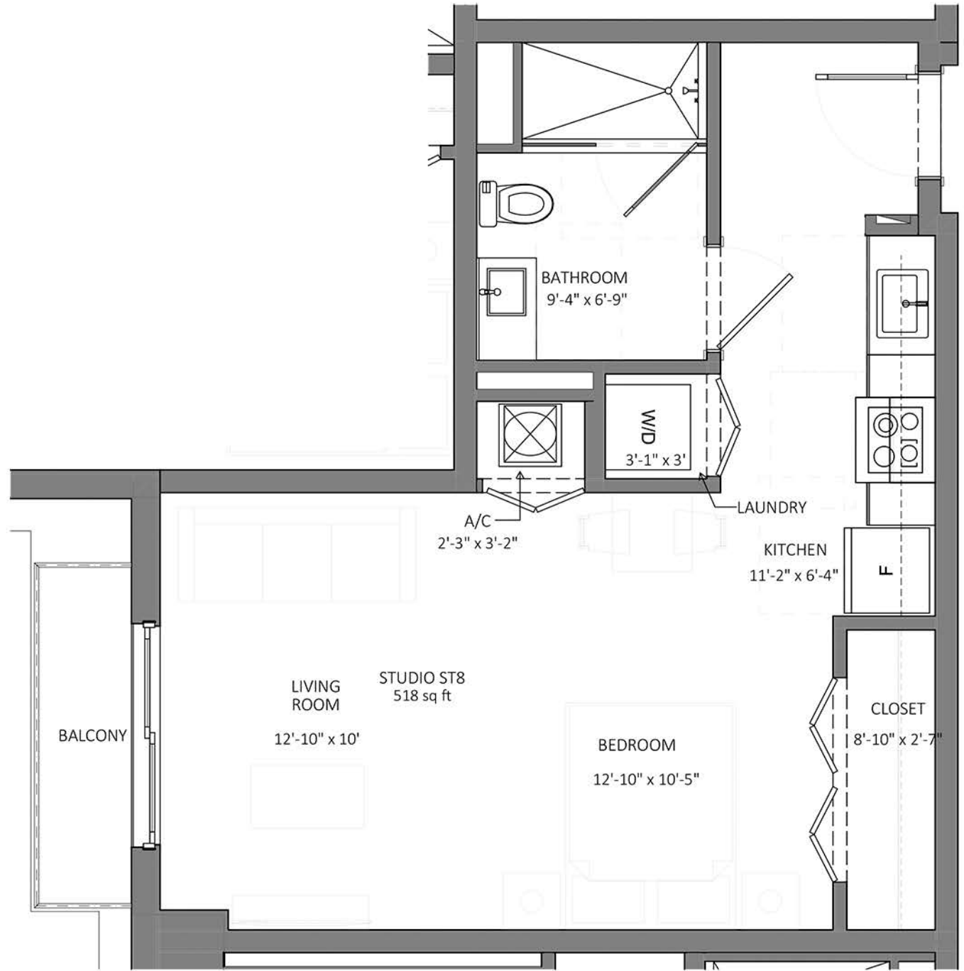
ST8 STUDIO UNIT ST8 SCALE: 1/4" = 1'-0"
